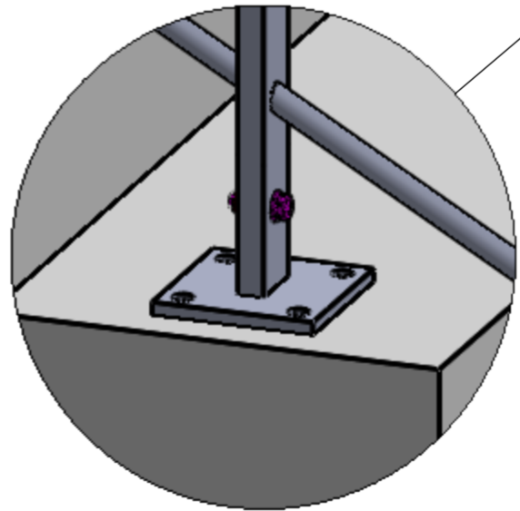
DÉTAIL H ECHELLE 1 : 4
