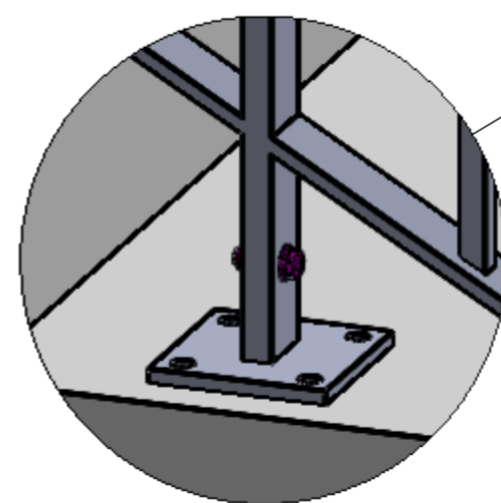
DÉTAIL M ECHELLE 1 : 4
