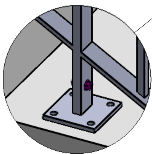
DÉTAIL A ECHELLE 1 : 4
