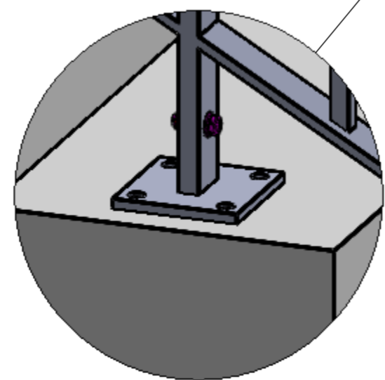
DÉTAIL C ECHELLE 1 : 4
