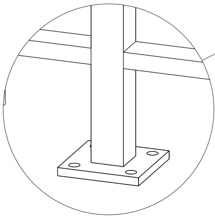
DÉTAIL B ECHELLE 2 : 5
