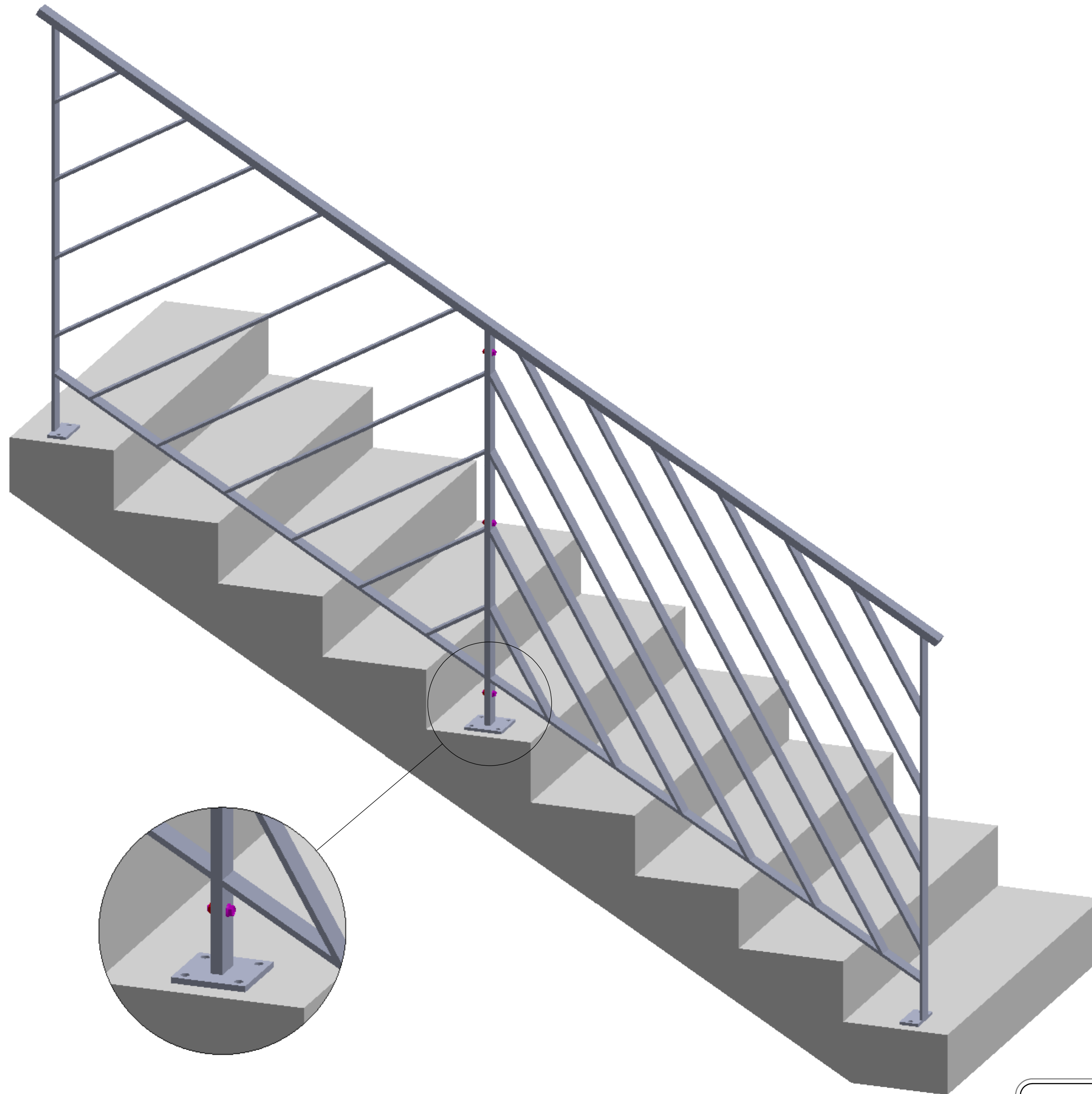
DÉTAIL Q ECHELLE 1 : 4
