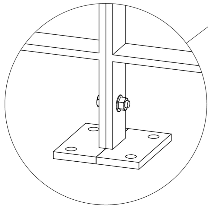
DÉTAIL A ECHELLE 2 : 5
