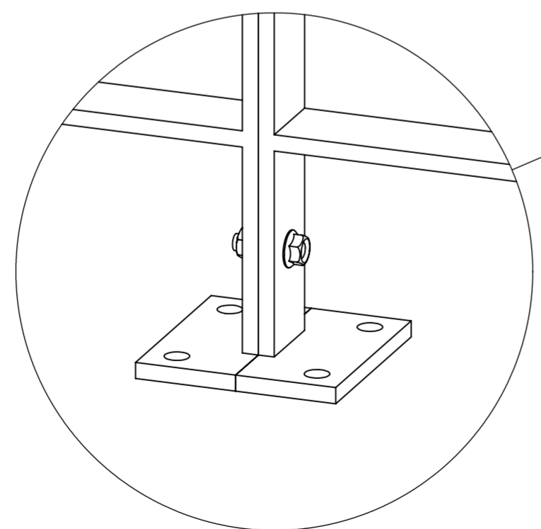
DÉTAIL A ECHELLE 2 : 5
